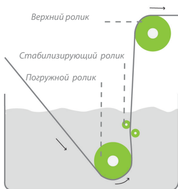
Схема ванны для расплавления цинкового сплава (цинковый котел)
